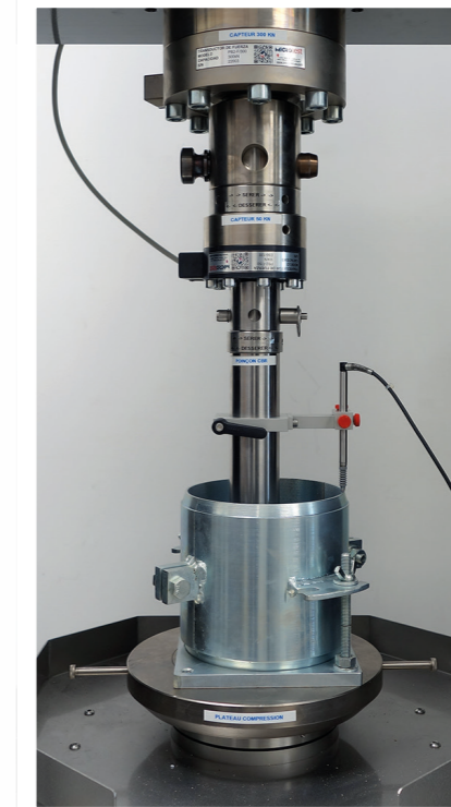
DISPOSITIF DE POINÇON / CBR
