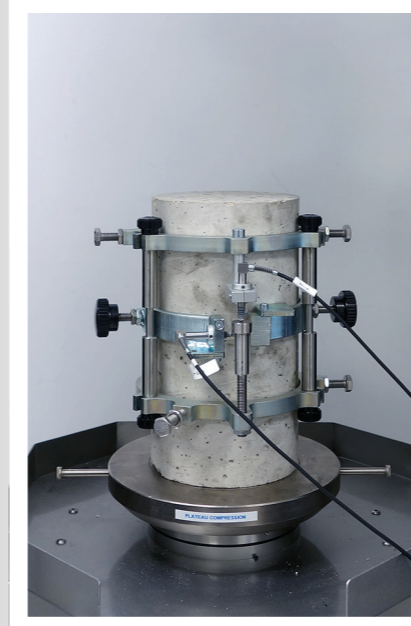
EXTENSOMÈTRE LONGITUDINALE
